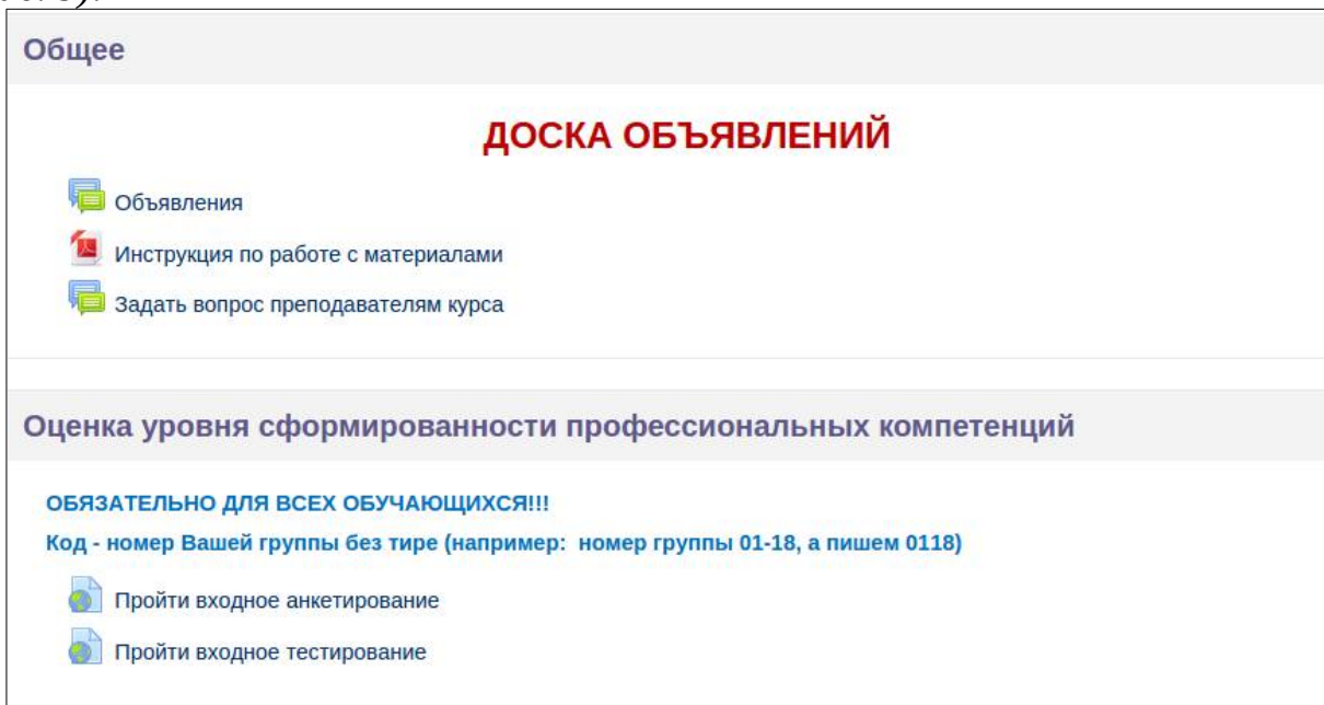
Рис. 9. Страница курса.
