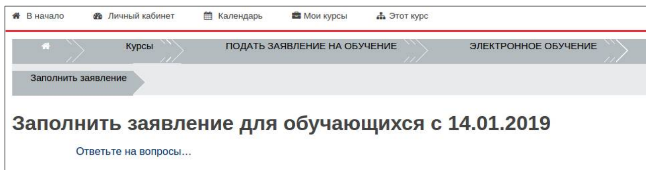
Рис. 6. Заполнение заявления.
